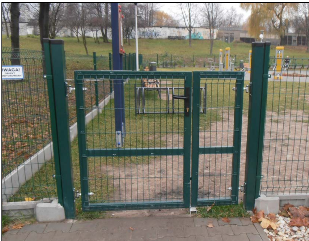
Fot.6 Projektowana furтка dwuskrzydłowa - niesymetryczna (skrzydła szerokości 1,0 i 0,5m, wysokość 1,2m).
